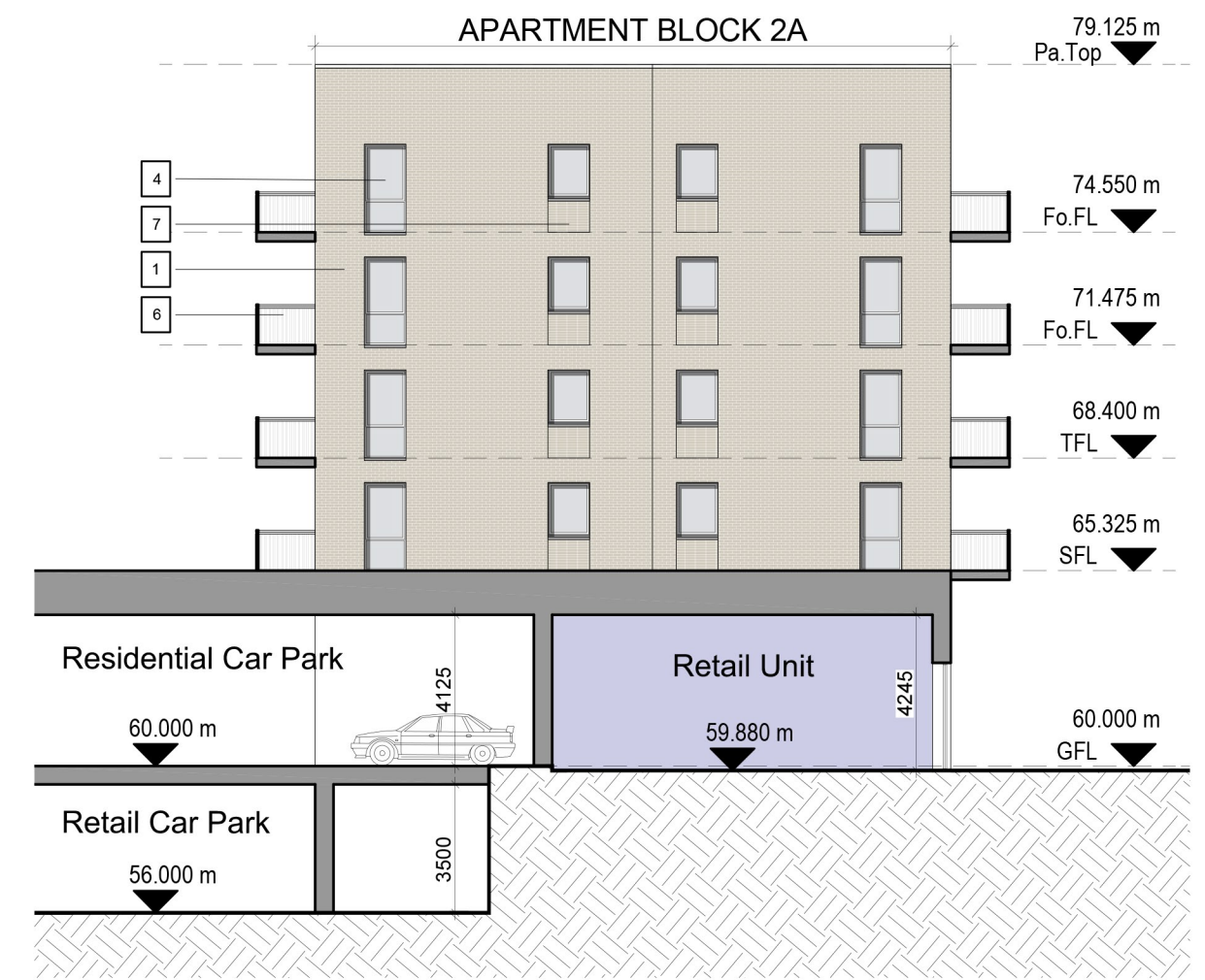
F Site Section FF 1 : 200
