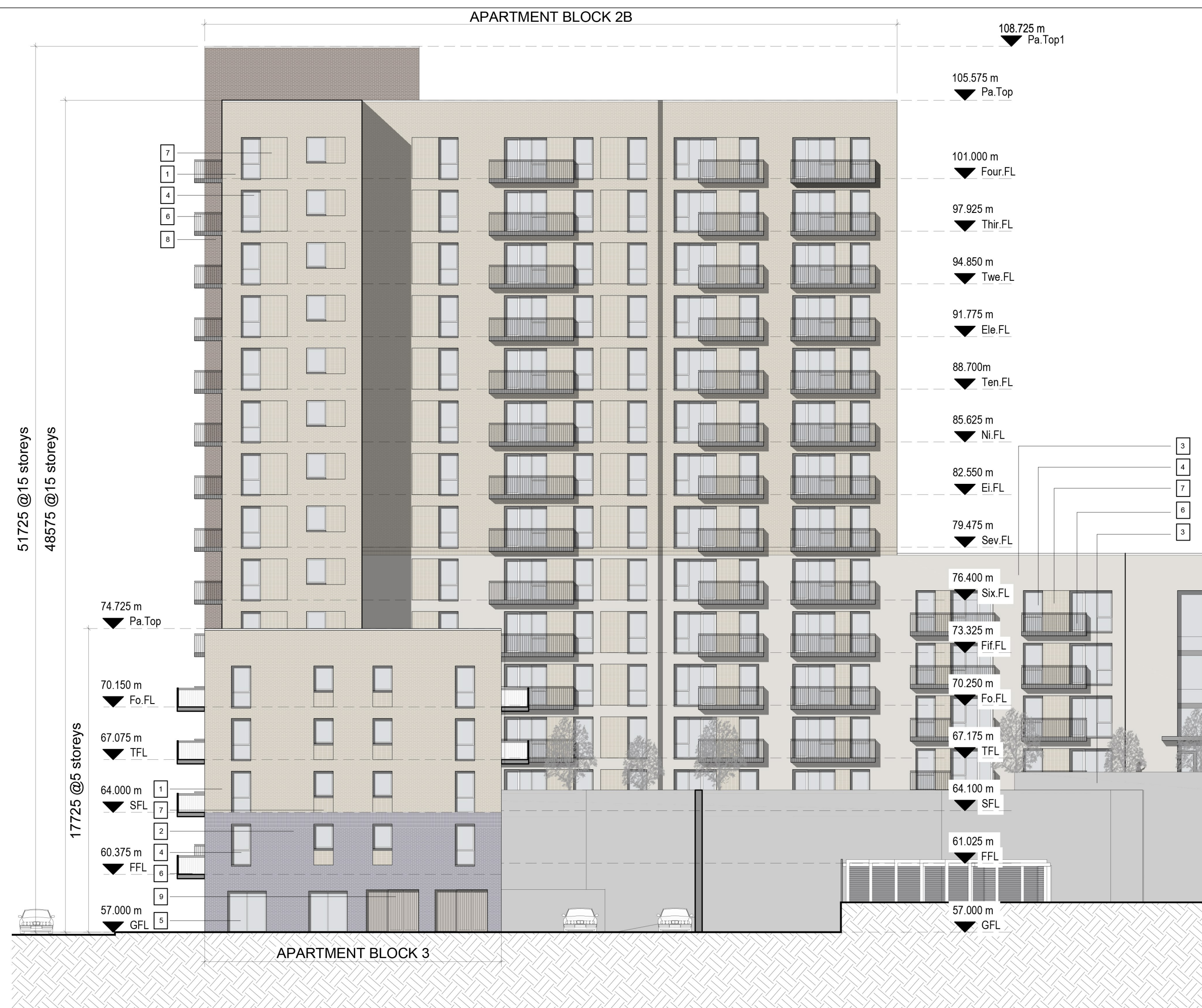
C Site Section CC 1 : 200
