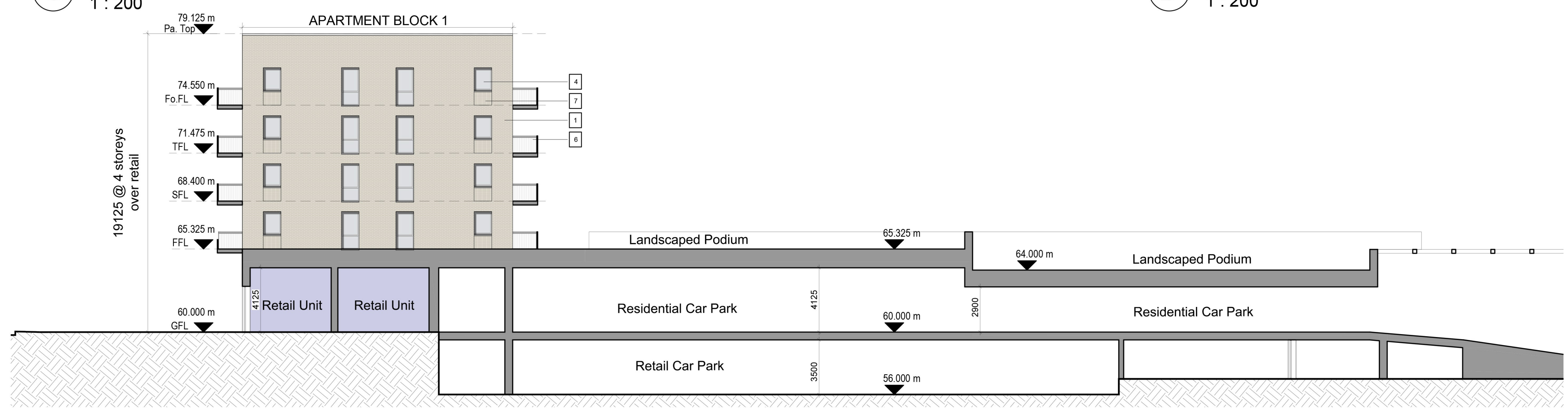
E Site Section EE 1 : 200
