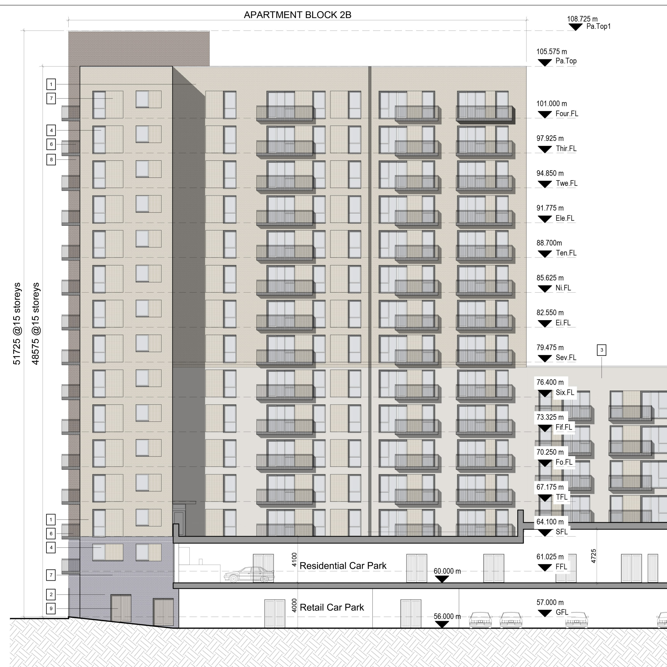
D Site Section DD 1 : 200
